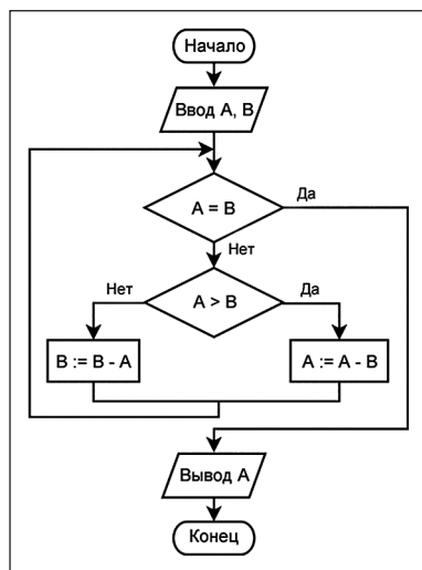
Алгоритм Евклида 1
